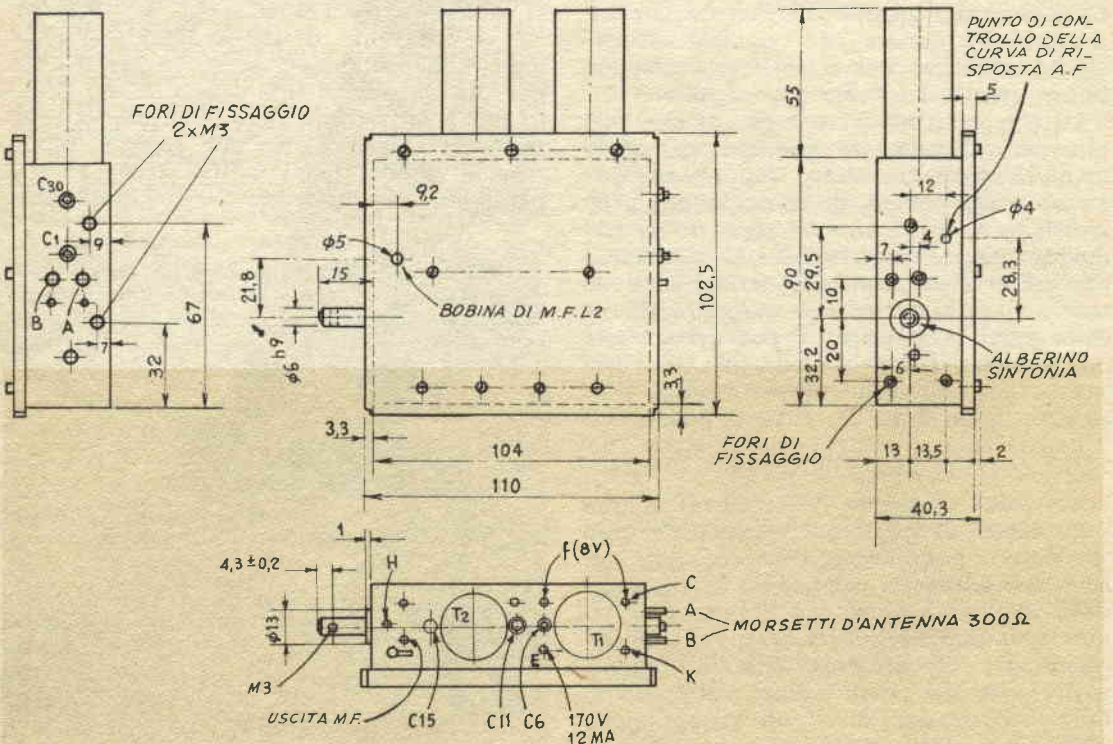
DATI D'INGOMBRO IN mm DEL SELETTOR AT 6321/38
