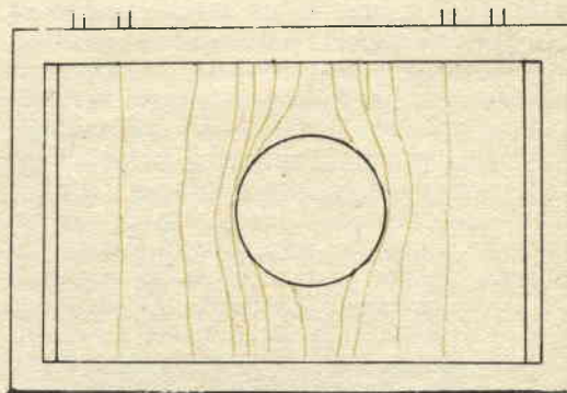
Ecco come si presentano, rilevati nel bagno elettrochimico, le linee che riproducono fedelmente i filotti fluidi del mezzo che viene attraversato dal modello, nel nostro caso un cilindro.
